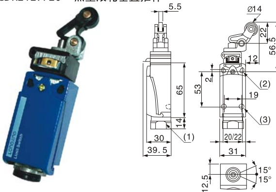
LL3XCDR2127P20 热塑滚轮垂直推杆
