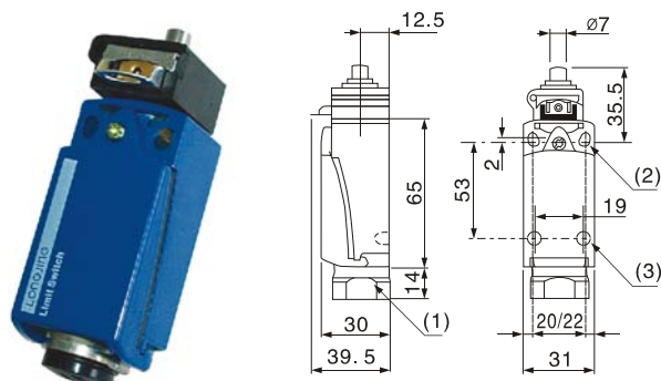
LL3XCDR2110P20 直动式
