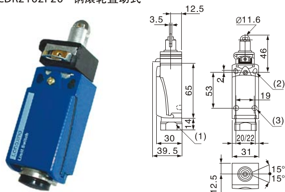
LL3XCDR2102P20 钢滚轮直动式
